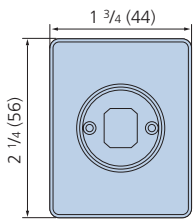
XCL-U1000/XCL-U1000C
