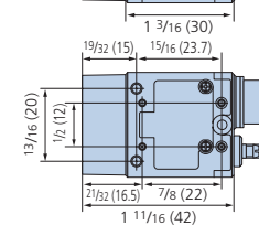
XCL-V500/XCL-X700
